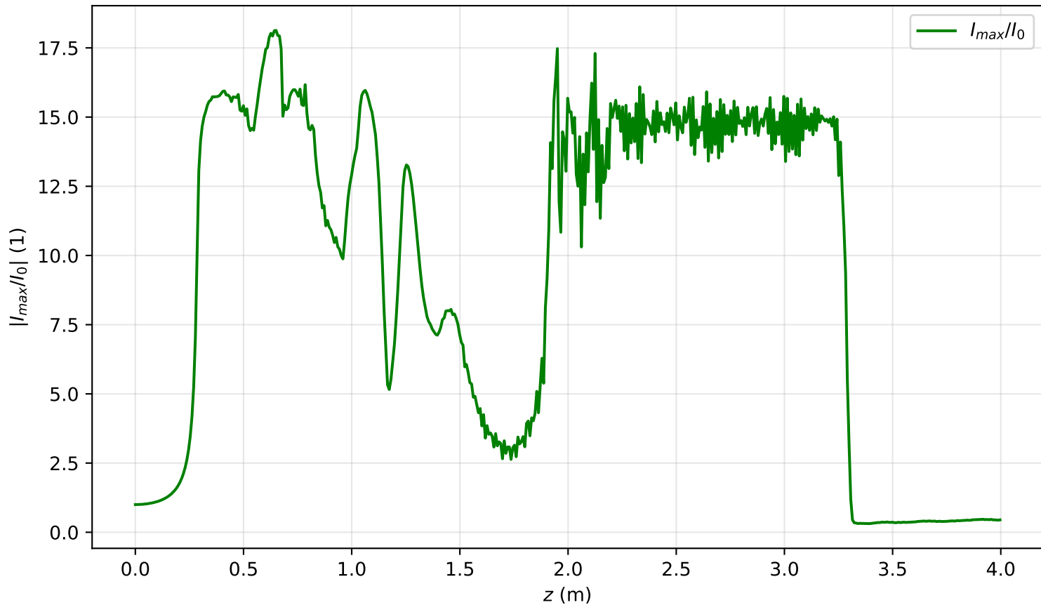
I_{\max}(r=0, z)/I_0 , Pin=9.9Pcr
